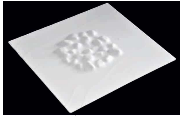
Rocas centrales
